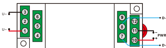
RS-485接线图:
